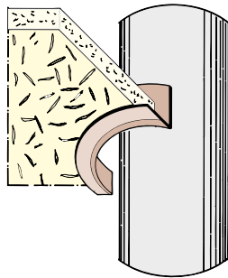
Anschluss an Rundstütze (konvex)
